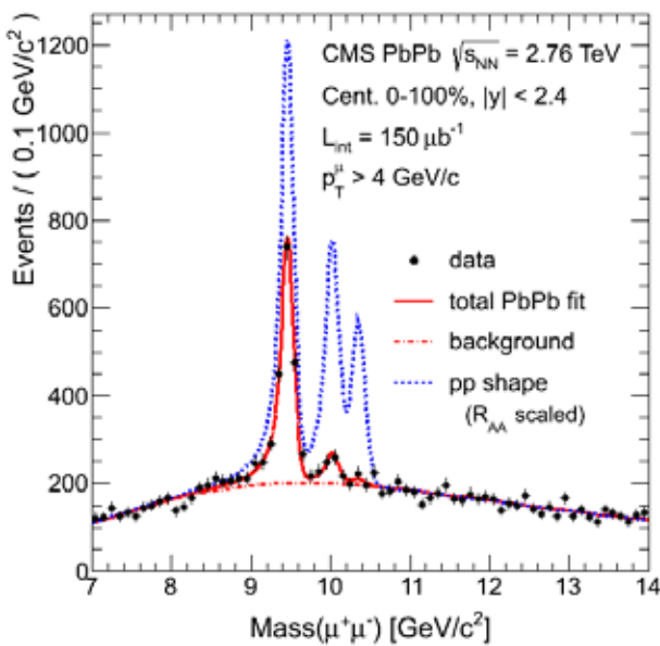
Suppression des upsilon, en rouge et noir les taux observés en collisions PbPb, en bleu les taux extrapolés.
